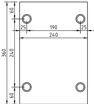
CONDUIT LOCATION BOX BASE
